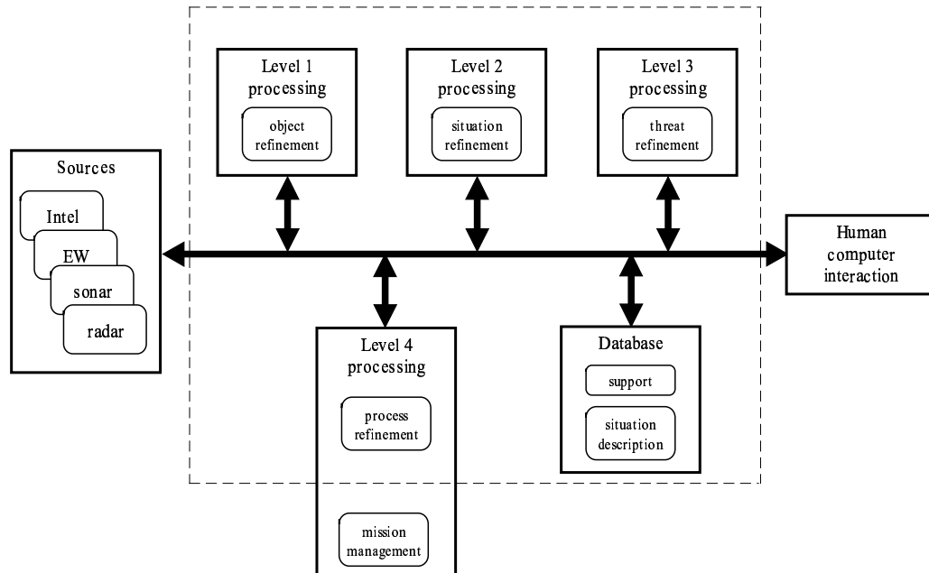
FIG. 5.1. : Modèle fonctionnel de la fusion de données selon [ANT95]
