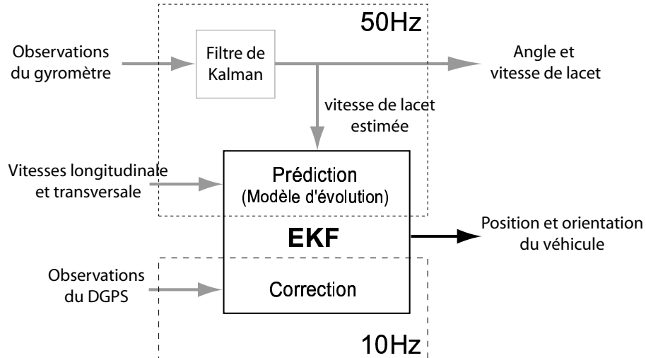
FIG. 5.11. : Architecture du module de positionnement
