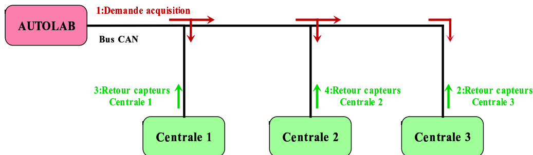
FIG. 6.8. : Principe de communication maître/esclave
