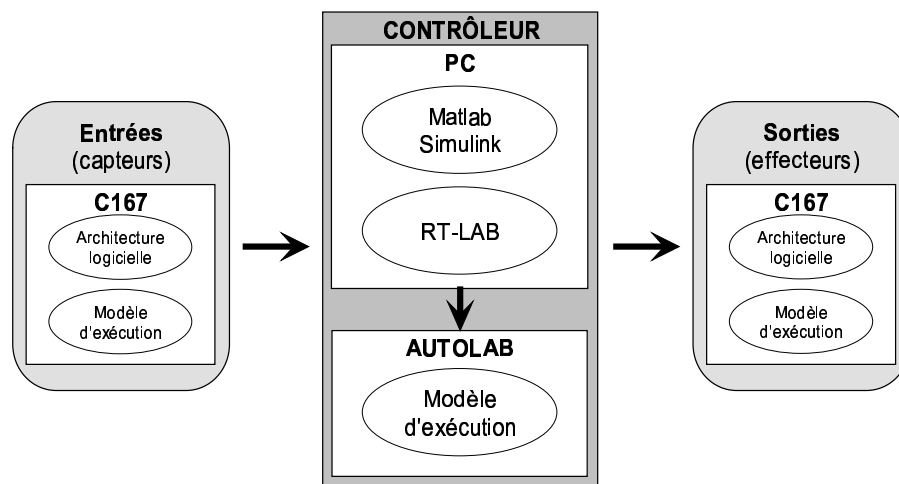
FIG. 6.9. : Architecture d'exécution
