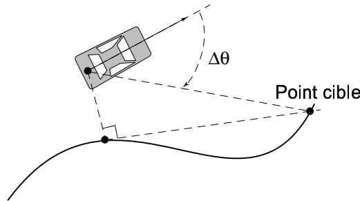
FIG. 3.21. : Technique de poursuite de cible
