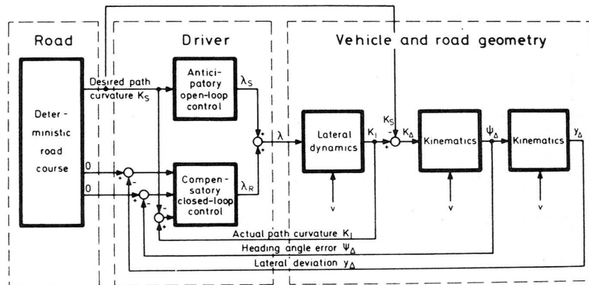
FIG. 1.6. : Le modèle conducteur à deux niveaux selon [DON78]
