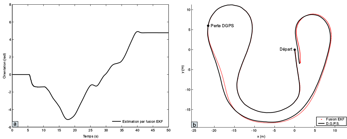
FIG. 6.17. : Fusion des informations par EKF
