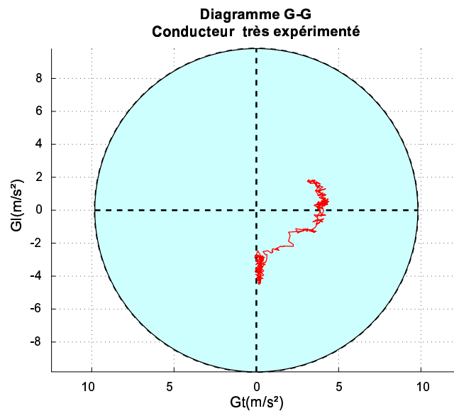
FIG. 3.12. : Diagramme G-G : virage 14
