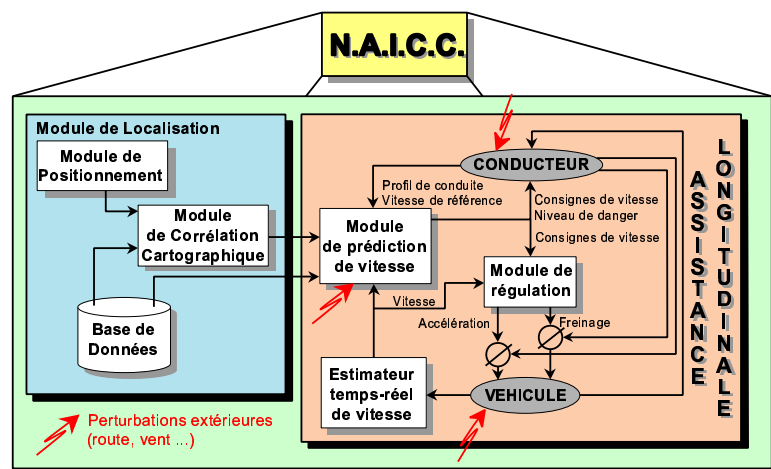
FIG. 2.8. : NAICC : l'assistance longitudinale
