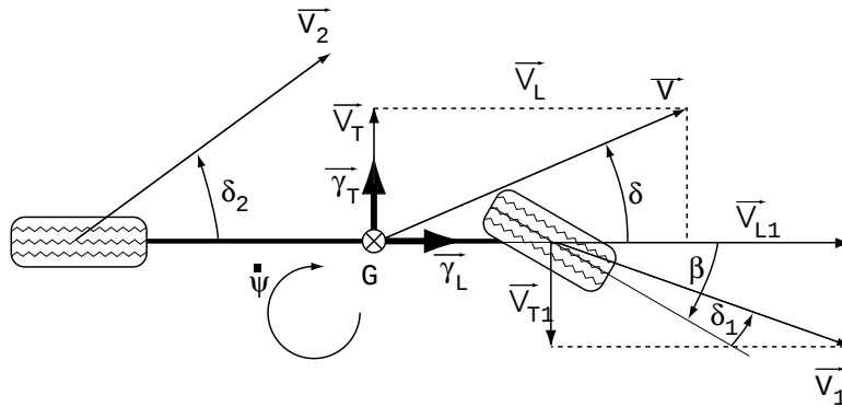
FIG. 1.2. : Modèle “lacet-dérive”
